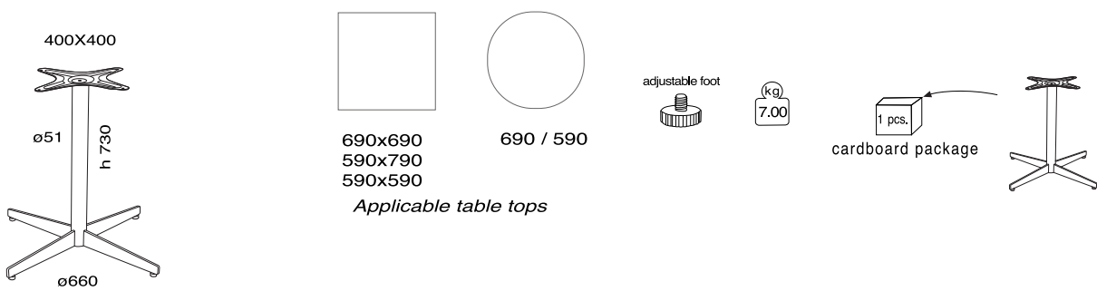
Gala 343 Bar Table base
