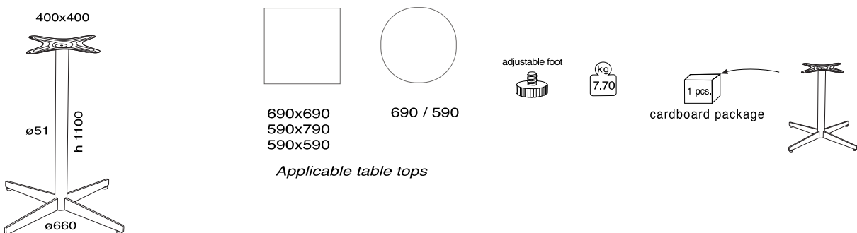
Gala 343 Bar Table base
